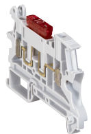
Bloc réf. 371 80 avec fusible automobile à languette
