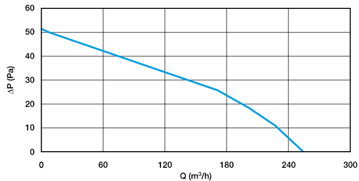
Courbe aéraulique GRAPHIC 125
