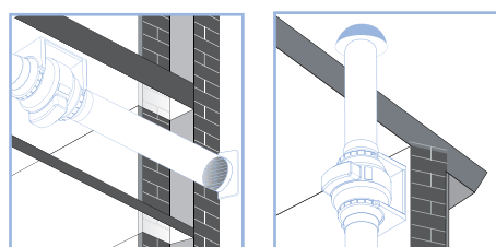
Montage horizontal
