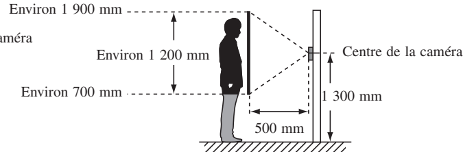
Position de montage 1 300 mm
