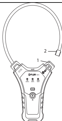
Fig. 5-2 Verrouillage des mâchoires de la pince
