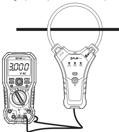
Fig. 5-1 Raccordement au DMM
