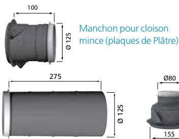
Manchon long
