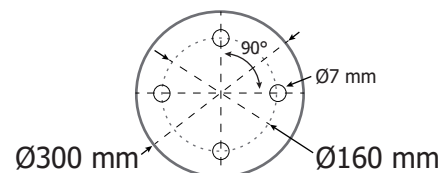
Schéma de pré-perçage de fixation
