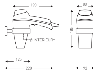
*Ø INTERIEUR DU SUPPORT MURAL : 80 MM
