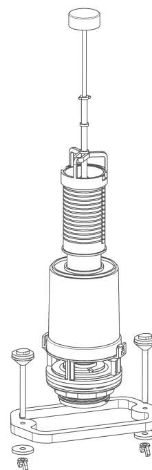
Adapté aux dimensions du réservoir ASPIRAMBO PORCHER
