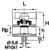
Vanne pour sondes à montage direct
