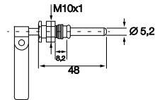
Sonde à montage direct (compatible EN1434)
