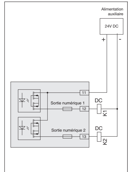
Fig. : Exemple de deux relais électroniques connectés aux sorties numériques
