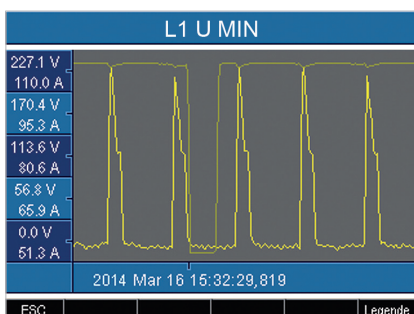
Fig. : Illustration des valeurs effectives pleine onde pour un événement (chute de tension)
