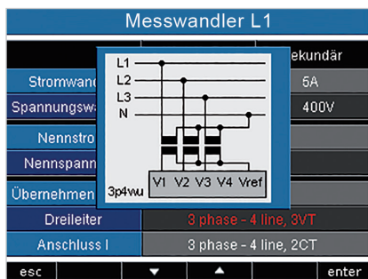
Fig. : Exemple de la configuration de la mesure du courant via trois transformateurs de courant dans un réseau tétraphasé sur l'écran de l'UMG 509.
