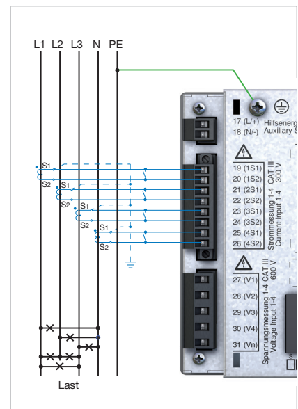
Fig. : Exemple de mesure du courant
