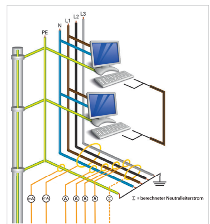
Fig. : Exemple de mesure RCM
