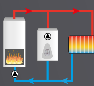
Chaudière bois
