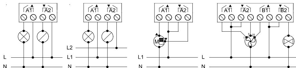
Figure 2: Exemples de connexions (de gauche à droite): 2 charges, 2 charges a phases différentes, volet roulant et ventilateur convecteur Fixer le MAXinBOX 24 sur le rail DIN:
