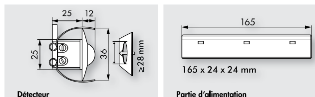
Détecteur
