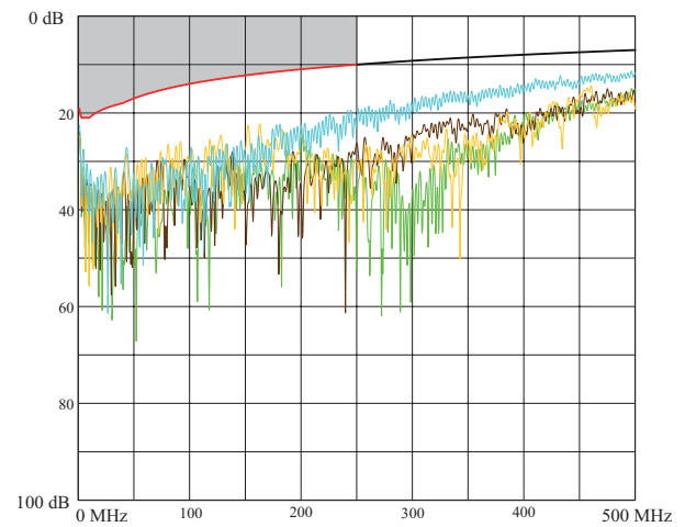
Return loss (Affaiblissement de réflexion)
