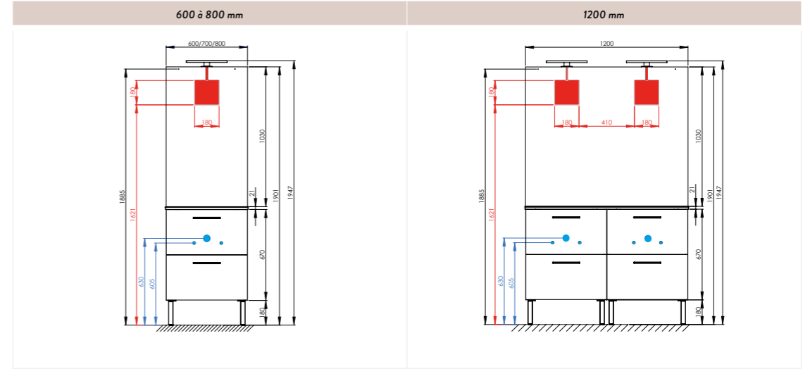
PLAN CÉRAMIQUE
