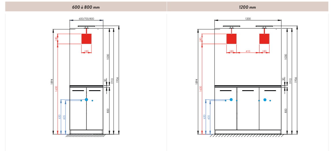
PLAN POLYBÉTON
