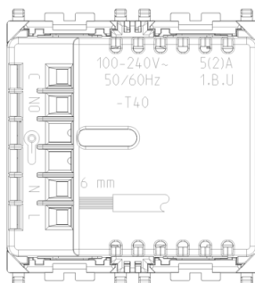
Vue arrière
