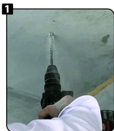
Percez Ø 8 mm (Ø16 à 20) Ø 10 mm (Ø22 à 26).
