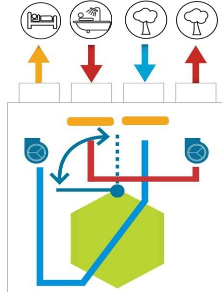
Fonctionnement avec By-pass
