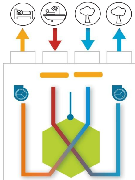
Fonctionnement sans By-pass
